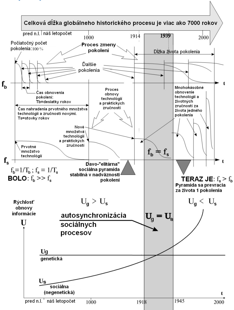
OBRAZ 6. ZMĚNA POMĚRU ETALONOVÝCH FREKVENCÍ BIOLOGICKÉHO A SOCIÁLNÍHO ČASU.
