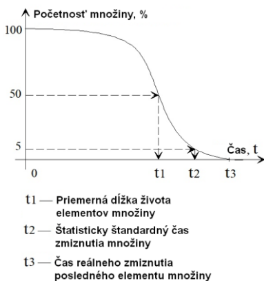
OBR. 5. CHARAKTER POSTUPNÉHO ÚBYTKU ELEMENTŮ Z PRVOTNÍHO SLOŽENÍ MNOŽINY
